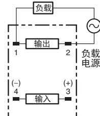
端子排布/内部连接 (顶视图)
