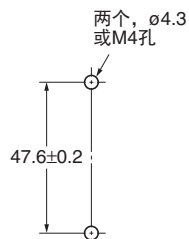
安装孔
