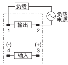
端子排布/内部连接 (顶视图)
